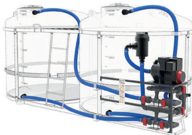
Комплекс насосный для СЗР/КАС на две емкости TRN 817л/мин d50мм ПВХ
