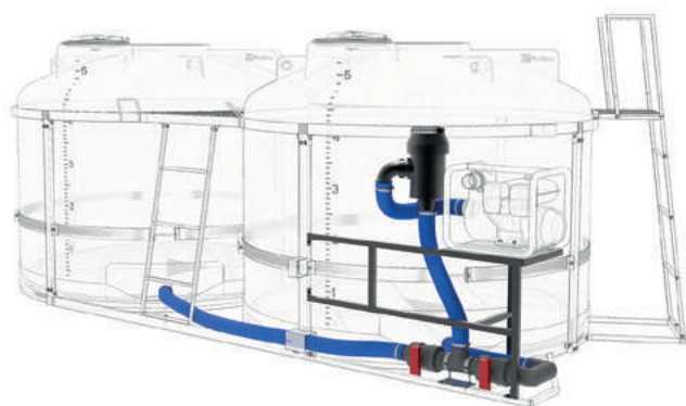
Комплект полного слива с фильтром и площадкой для мотопомпы на две емкости TRF d75мм PBX
