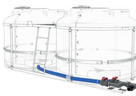
Комплекты слива с кранами - опорожнение емкостей.
