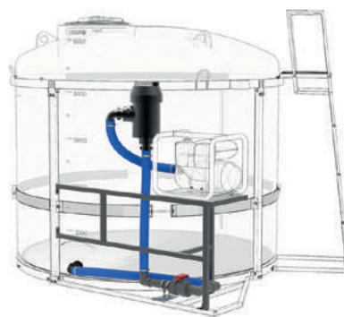
Комплект слива с фильтром и площадкой для мотопомпы на одну емкость TRN d50мм PBX
