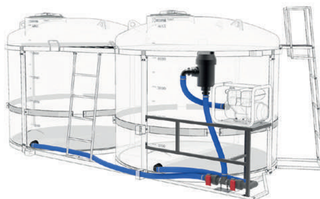
Комплект слива с фильтром и площадкой для мотопомпы на две емкости TRN d50мм PBX
